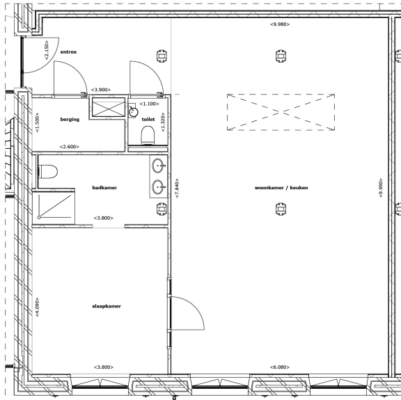
Plattegrond verdieping 01 1:50
